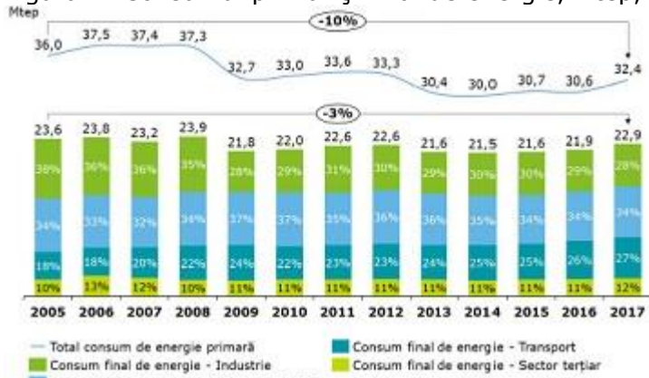
Figura 2: Consumul primar și final de energie, Mtep, inclusiv alocarea pe sectoare, 2005-2017
