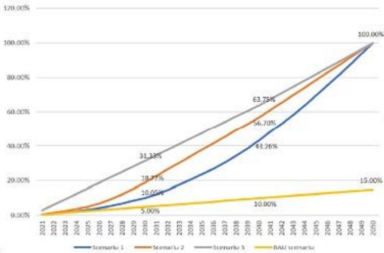
Ponderea de renovare cumulată a clădirilor în fiecare scenariu
